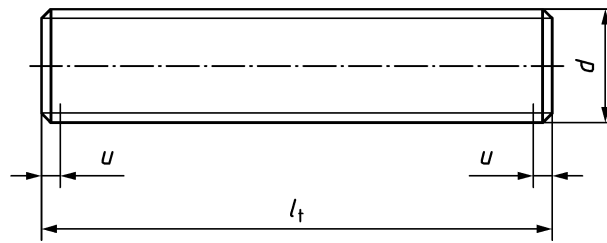
Bild 1 — Form A, Gewindeende RL nach DIN EN ISO 4753
